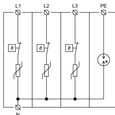
Vnútorná schéma zapojenia
